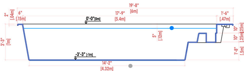
CORTE LONGITUDINAL | LONGITUDINAL SECTION | SECTION LONGITUDINALE
