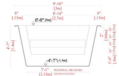
CROSS SECTION B-B SECCIÓN TRANSVERSAL B-B
