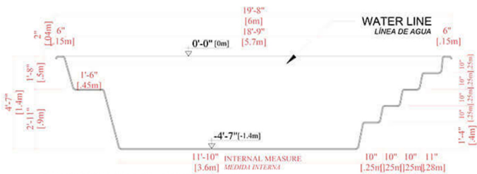
LONGITUDINAL SECTION A-A SECCIÓN LONGITUDINAL A-A
