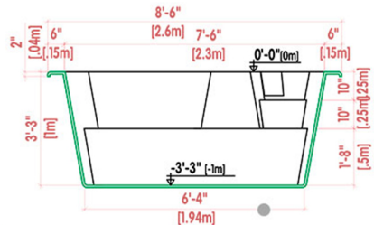
CORTE TRANSVERSAL | CROSS SECTION | LA COUPE TRANSVERSALE
