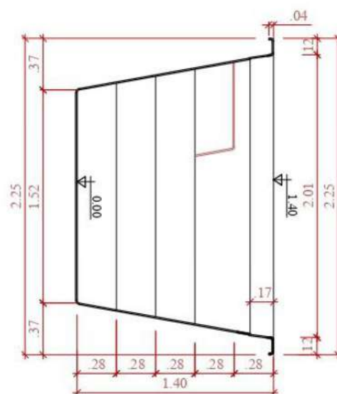
CORTE TRANSVERSAL SEM ESCALA
