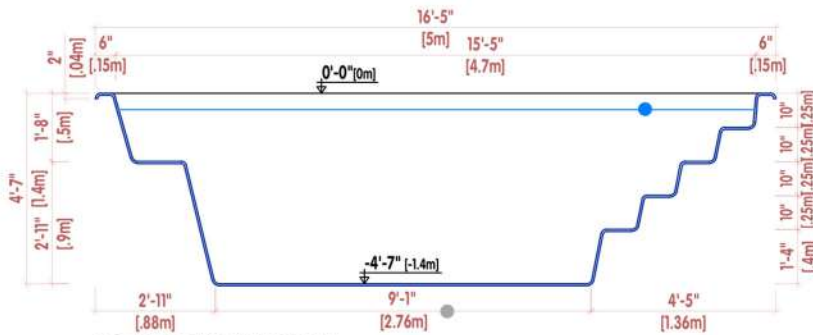
CORTE LONGITUDINAL | LONGITUDINAL SECTION | SECTION LONGITUDINALE
